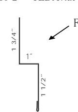
Ⓖ 29 Ga. Double Angle 10'2" TLDA7xx
