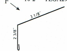
Ⓖ Gutter Apron 10'2" TLGA29xx
